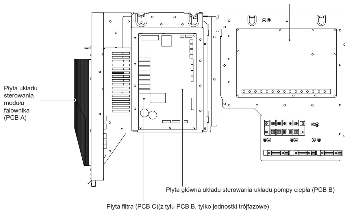
Płyta głównego układu sterowania modułu hydraulicznego
