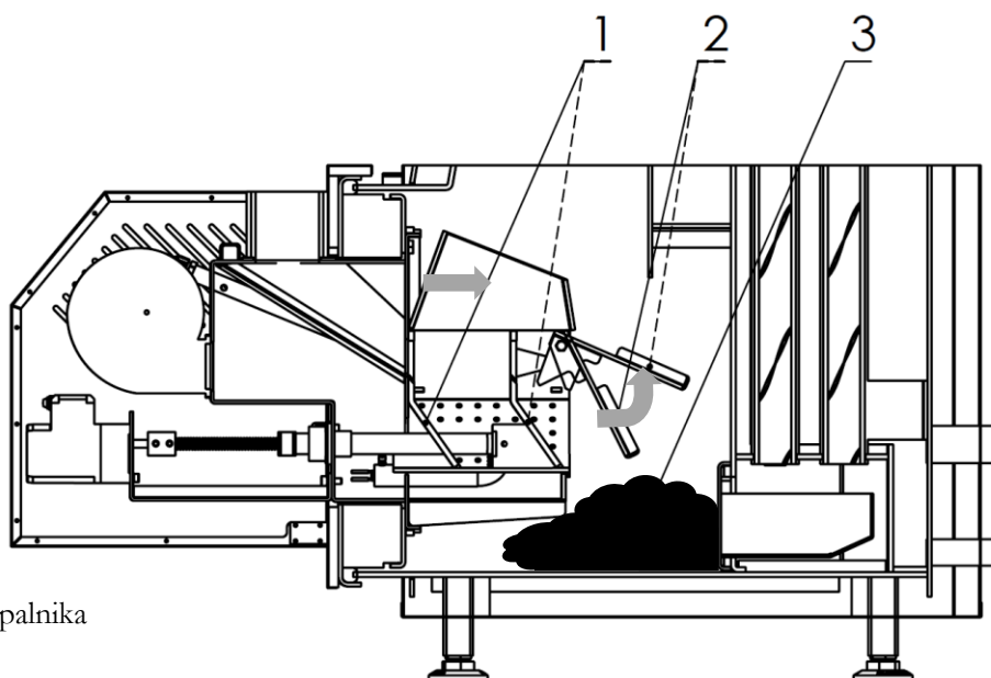
Rys. 23 Układu samoczyszczący palnika
