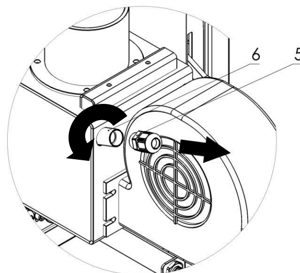
Rys. 20d. Wykręcenie dławicy
