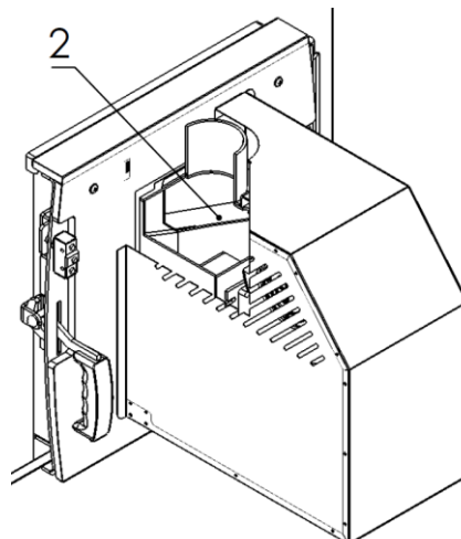
Rys. 22 Czyszczenie powierzchni spadu peletu
