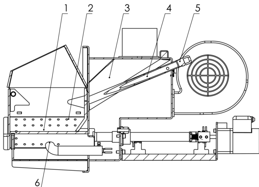
Rys. 20. Czyszczenie palnika
