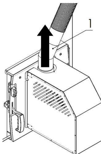
Rys. 22 Czyszczenie powierzchni spadu peletu
