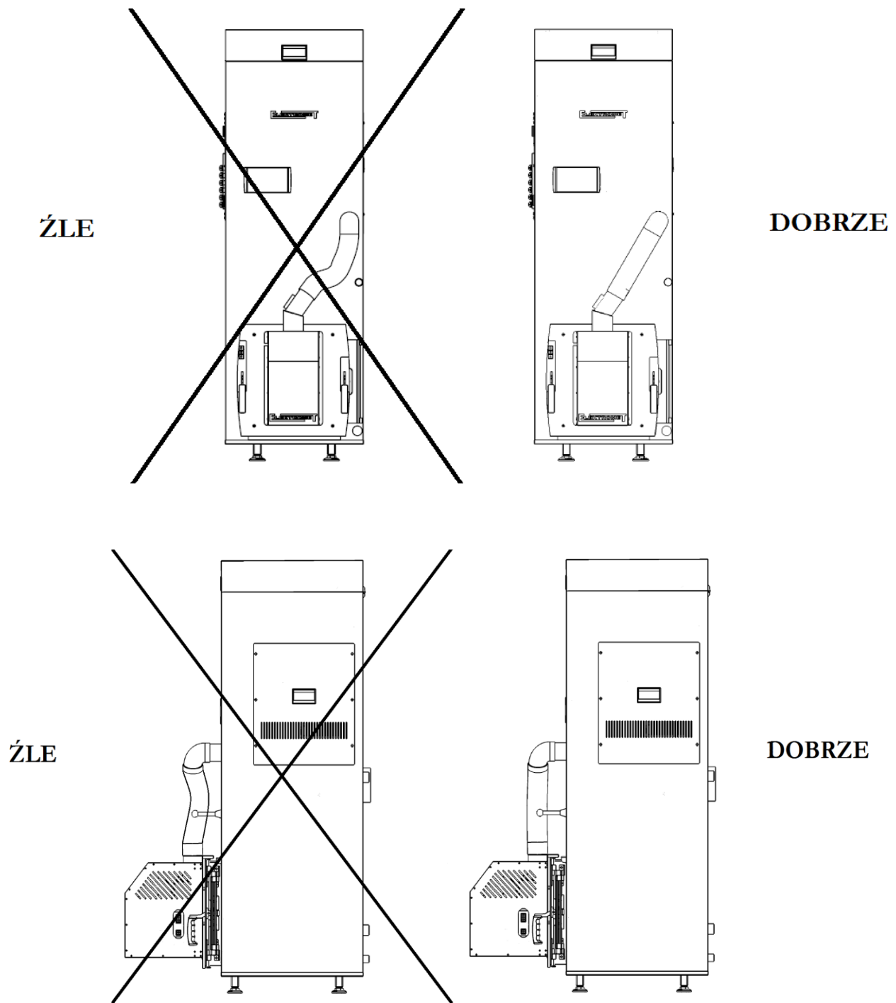
Rys. 6b. Prawidłowy sposób mocowania elastycznej rury zasypowej podajnika w kotle EKO-PE Compact.
