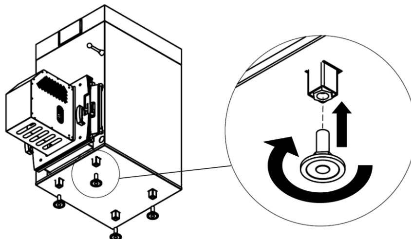
Rys. 4. Późimowanie kotła
