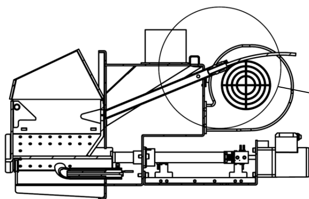
Rys. 21 Osadzenie czujnika
