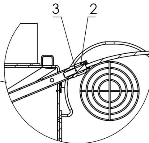
Rys. 20f. Czyszczenie rurki czujnika
