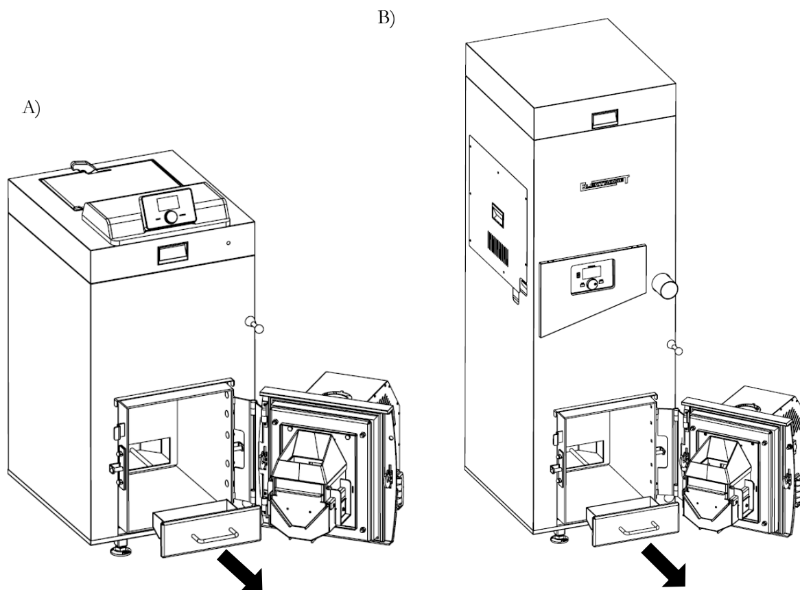
Rys. 19c. Czyszczenie tylnego popielnika kotła EKO-PE Compact w wersji: (A) - STANDARD oraz BOX, (B) - TOP
